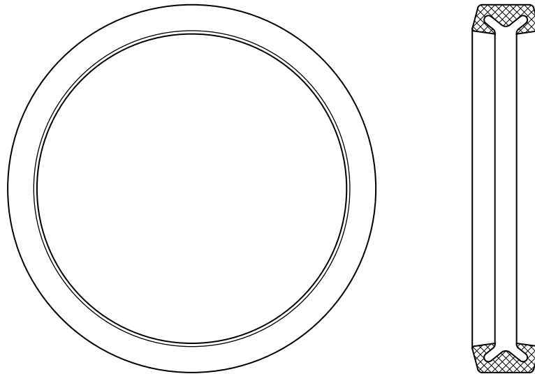
GUARNIZIONE IN GOMMA RINFORZATA – GG/R REINFORCED RUBBER GASKET
